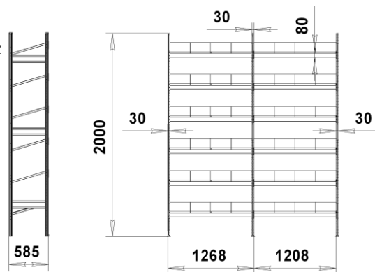
Схема вариантов установки СТ-023 Стеллаж наклонный
